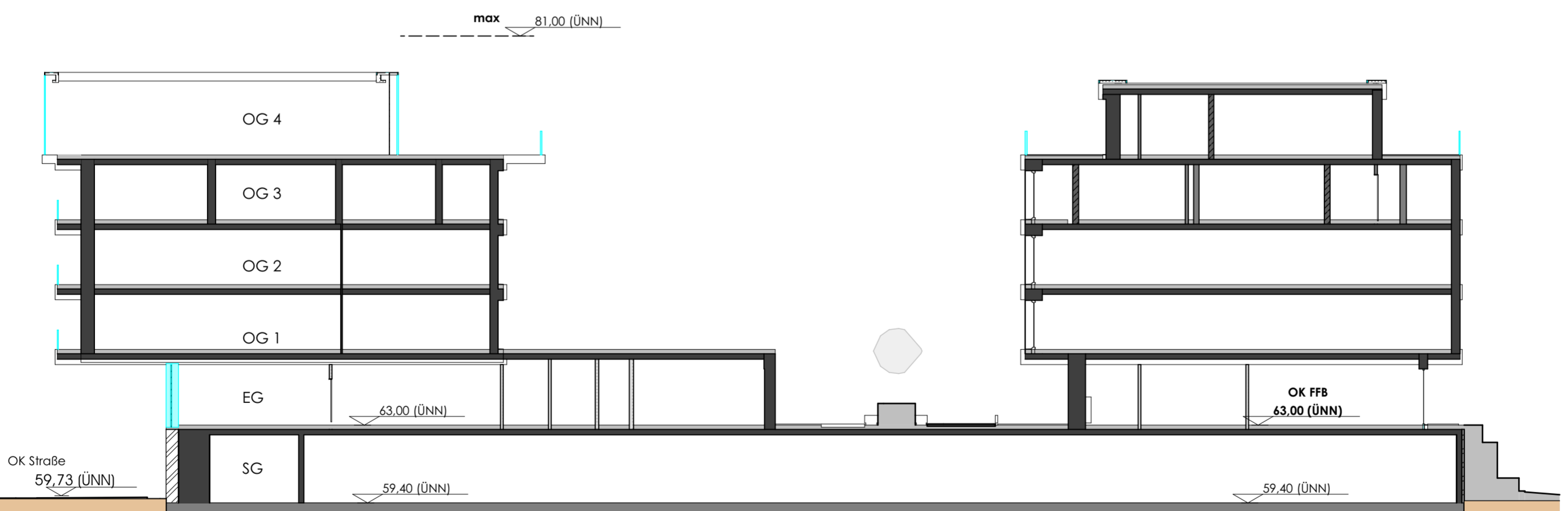
Schnitt A1 durch Haus 1 (Hotel) und Haus 2
