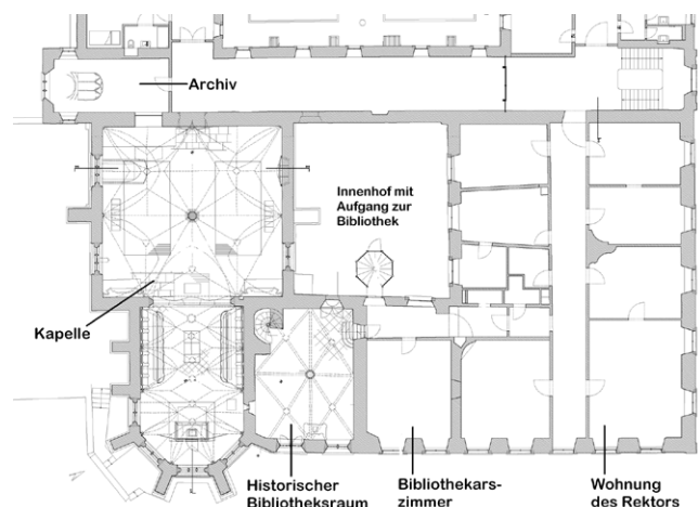
Grundriss Ostflügel des St. Nikolaus-Hospitals. Entwurf: Dipl.-Ing. Michael Leonhardt, Trier
