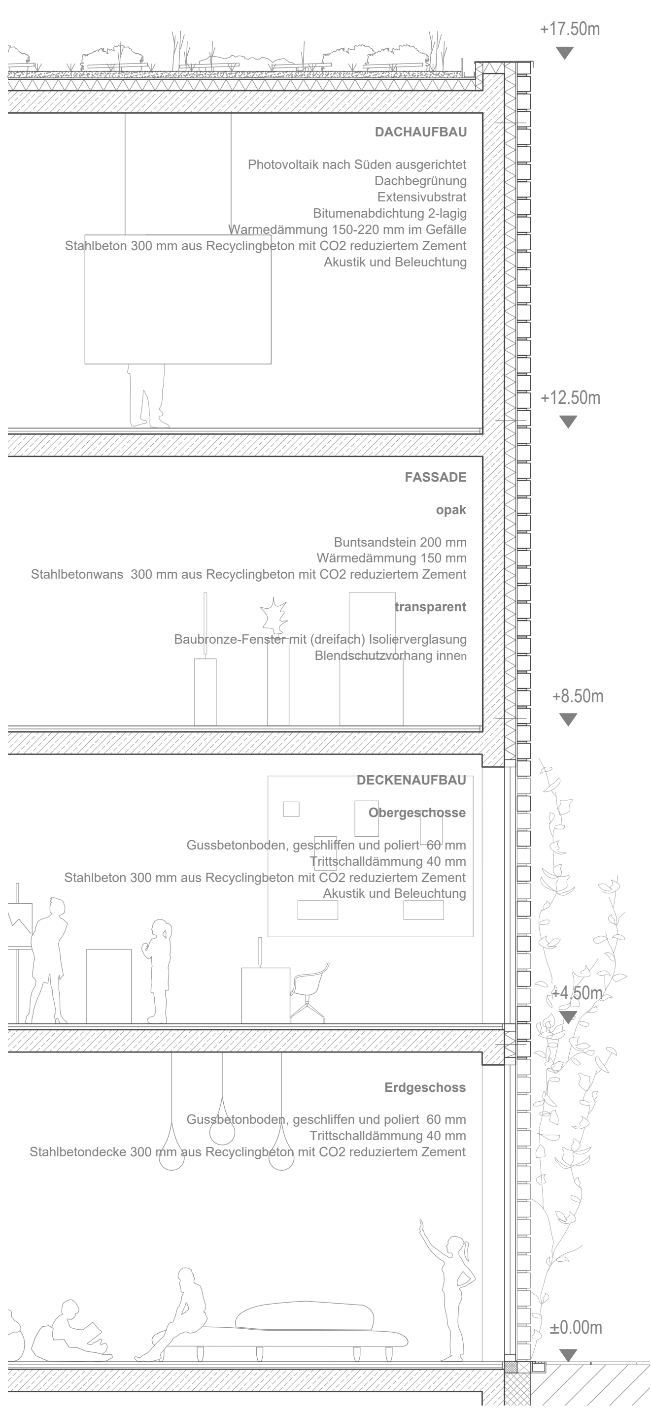
f Fassadenschnitt 1:50
