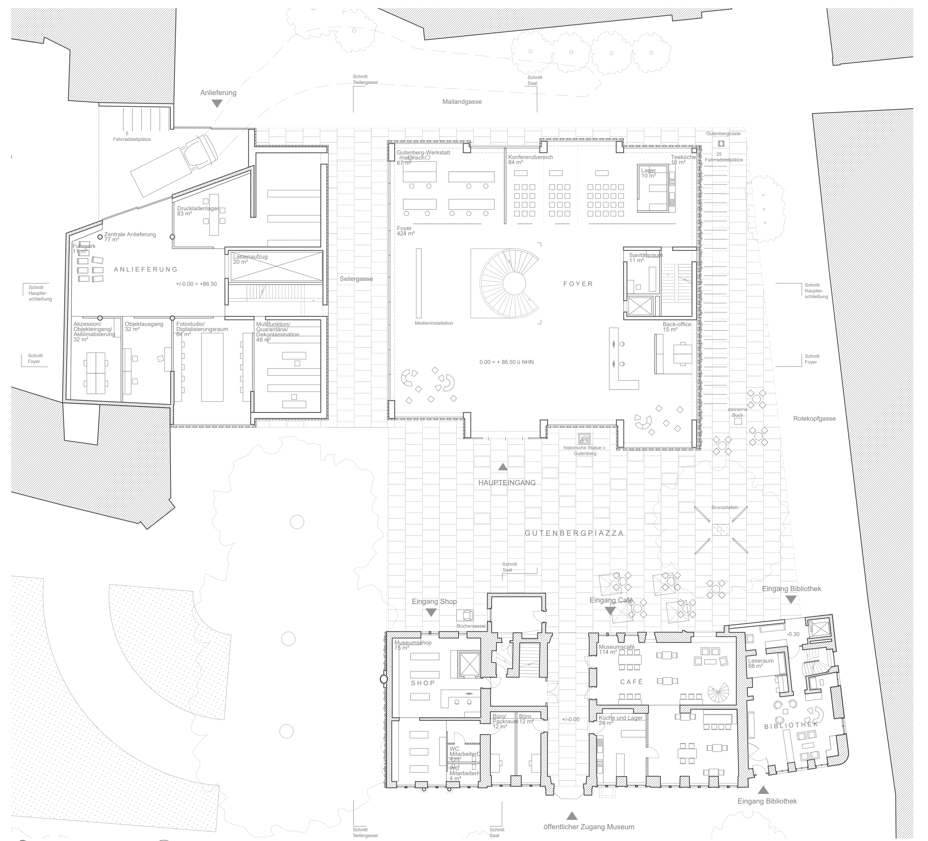
Erdgeschoss 1:200
