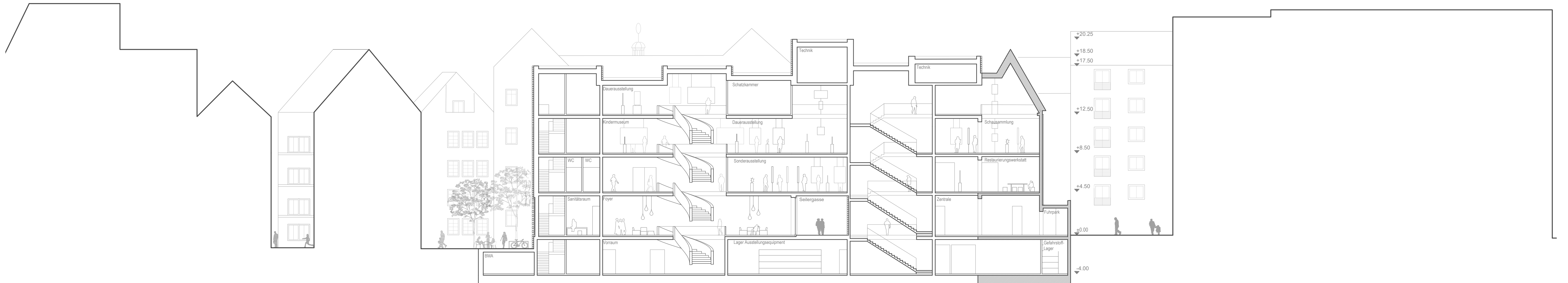
Schnitt Hauptschließung 1:200
