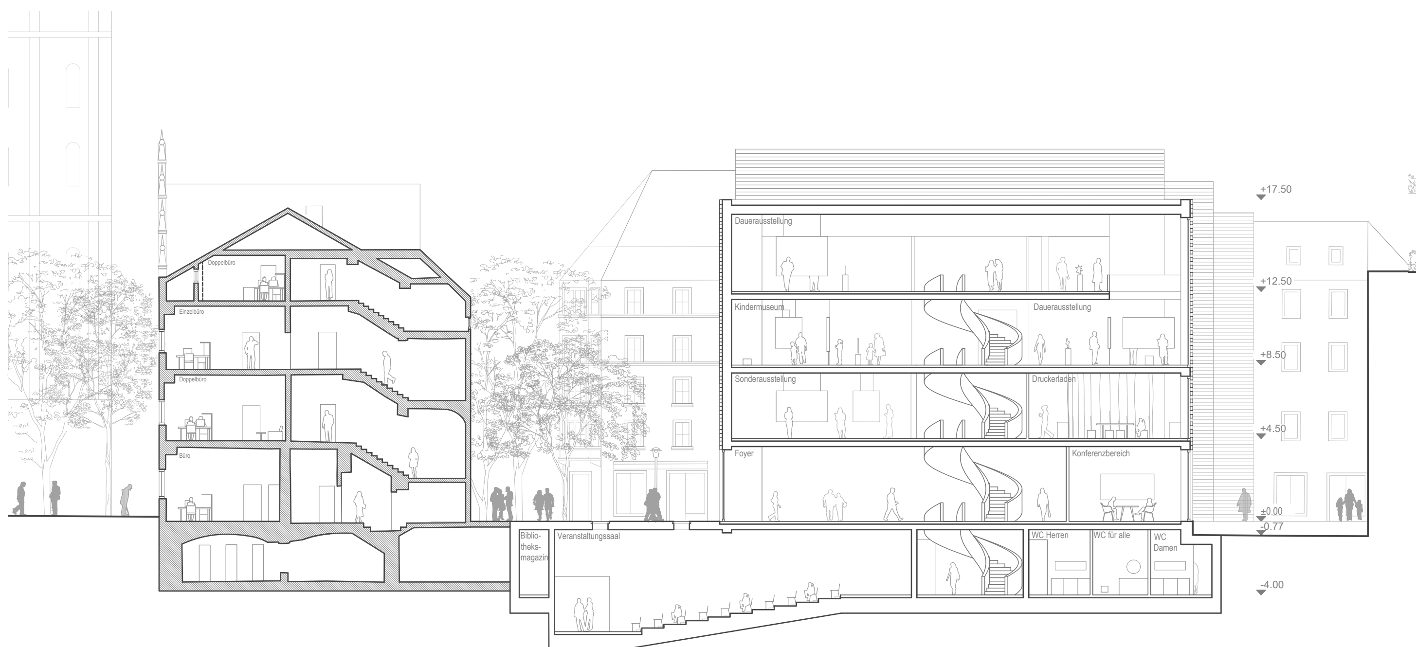
Schnitt Saal 1:200
