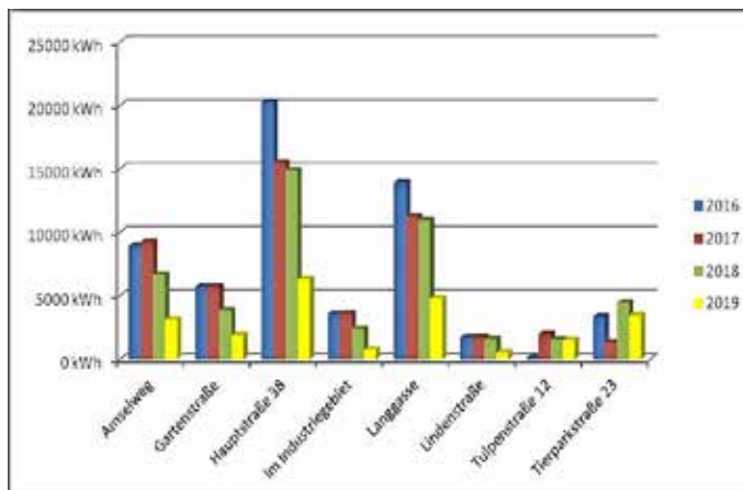
Stromverbrauch Straßenlampen
