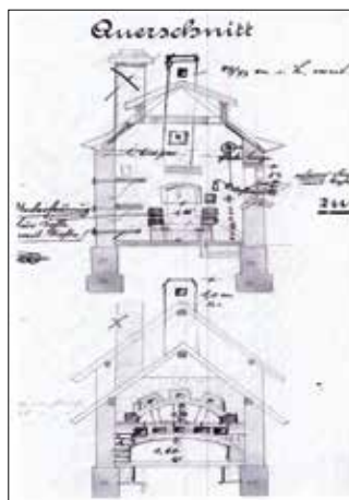
„Auszug aus dem historischen Bauplan von 1923“
