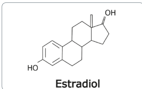
Chemische Struktur des Östrogens Estradiol
