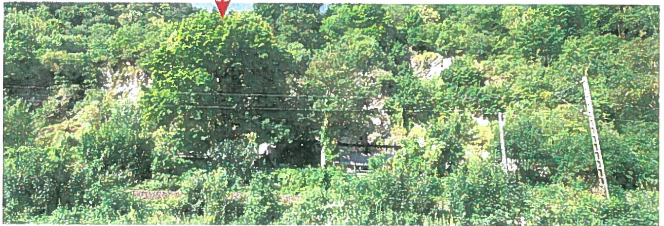
Detailfoto von Abschnitt A, im Hang tritt offene Felsbildung auf, ausbrechende Steine erreichen nicht das Gleis, da ausreichend Raum zwischen Hangfuß und Gleisanlagen vorhanden ist.
