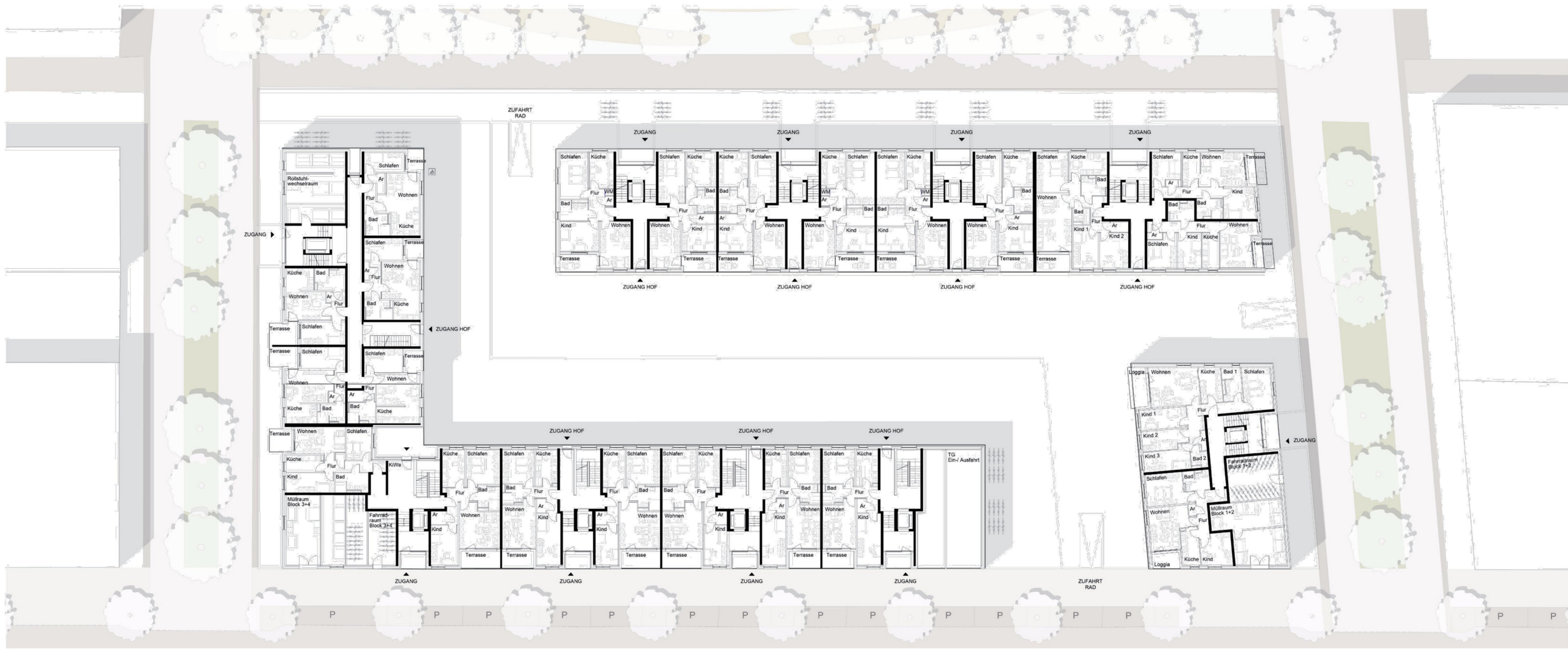
GRUNDRISS EG 1:200
