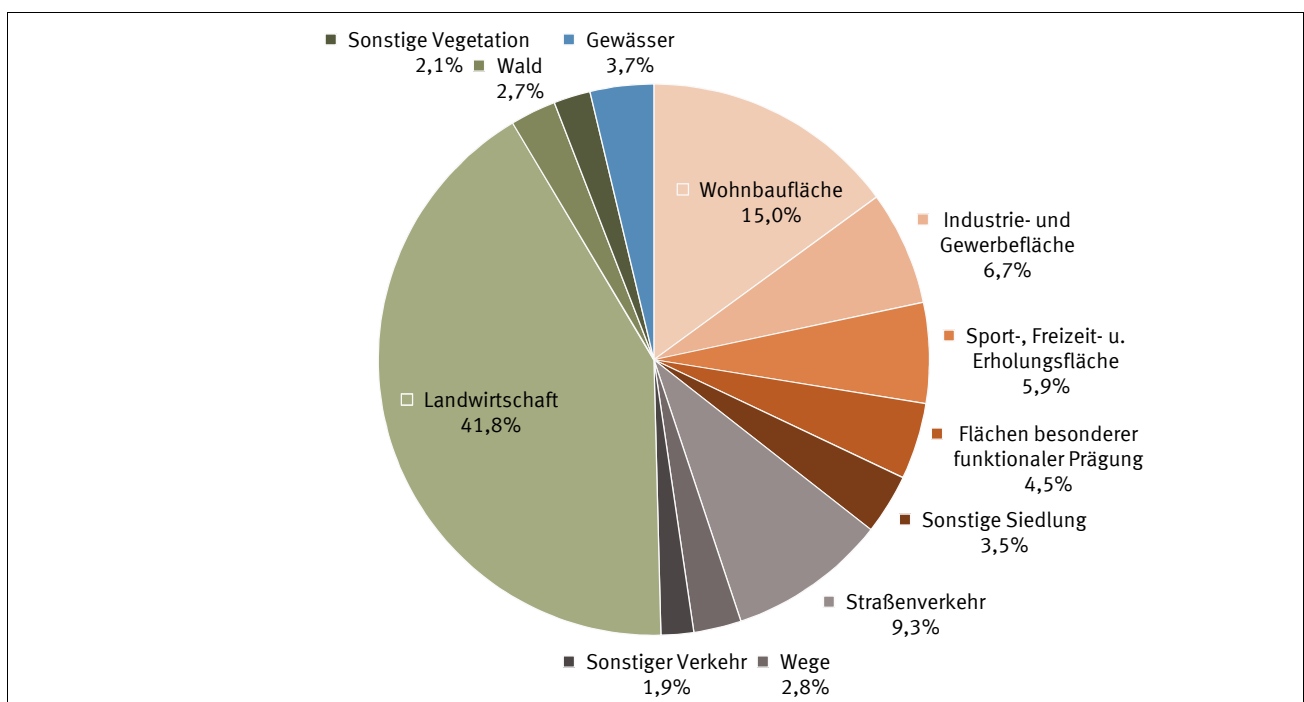
Abb. 1.1 Tatsächliche Flächennutzung 2020
