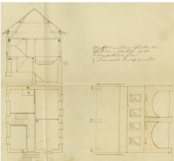
1856, Planzeichnung von Cyriak Weisrock II. zum Neubau von Veit Stauder, Pariser Straße Nr. 65. 46
