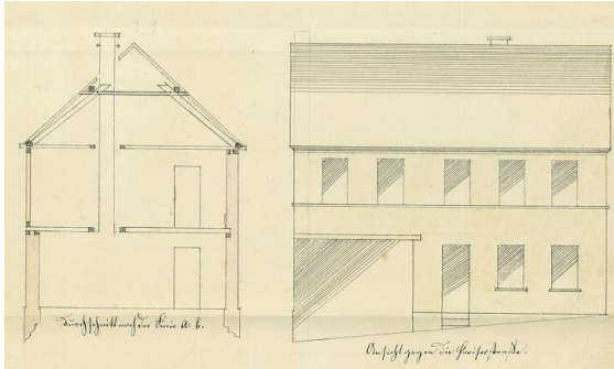
1863, Planzeichnung von Bernard Ruf II. zum Neubau von Caspar Wintersinger, Pariser Straße Nr. 115. 60
