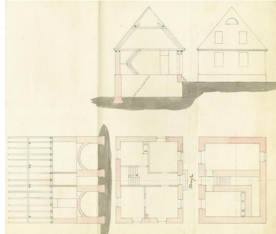
1868, Planzeichnung von Heinrich Weisrock zum Neubau der Wittve Horn. 48
