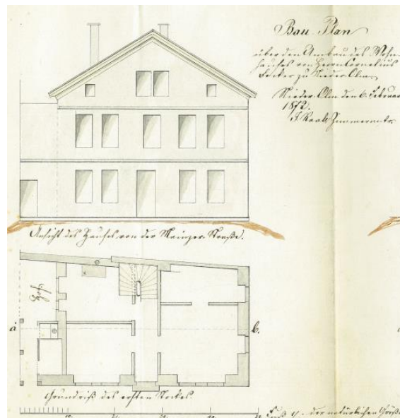
1872, Planzeichnung von Johann Raab zum Bauantrag von Cornelius Becker, Domherrnstraße Nr. 1. 65
