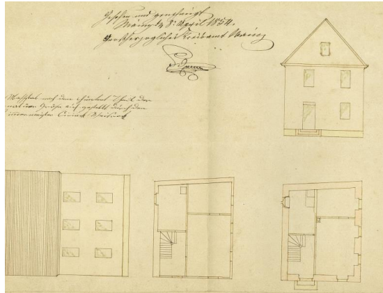
1856, Planzeichnung von Cyriak Weisrock II. zum Neubau der Postexpedition von Friedrich Koch, Pariser Straße Nr. 104. 45
