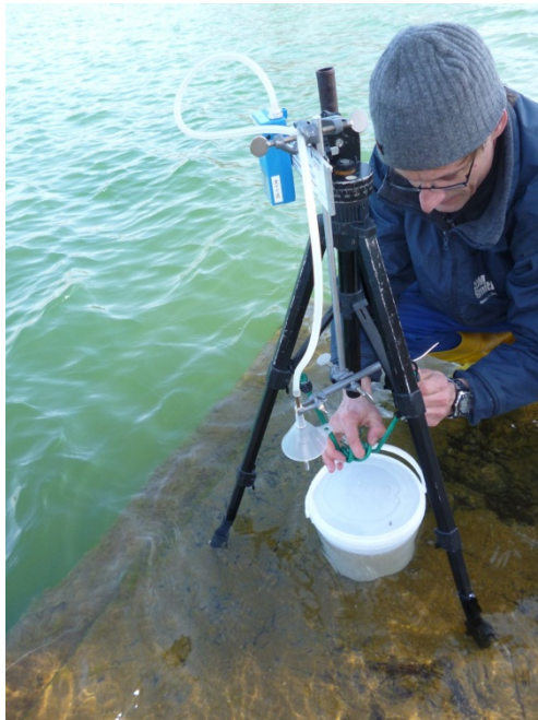
Foto Nr. 4: MP2 Bootanleger (Aufstellen Probenahmeapparatur)
