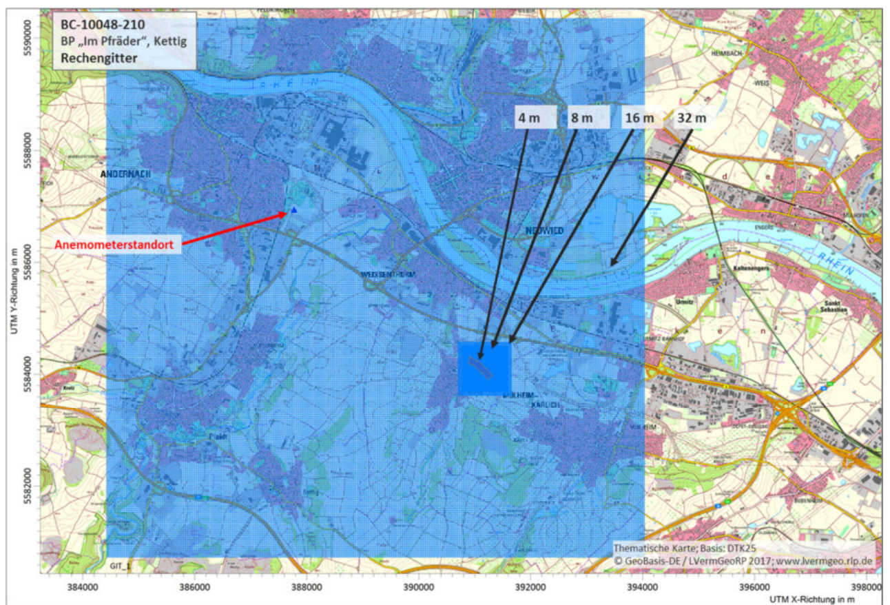
Abbildung 11: Rechengitter und Anemometerposition
