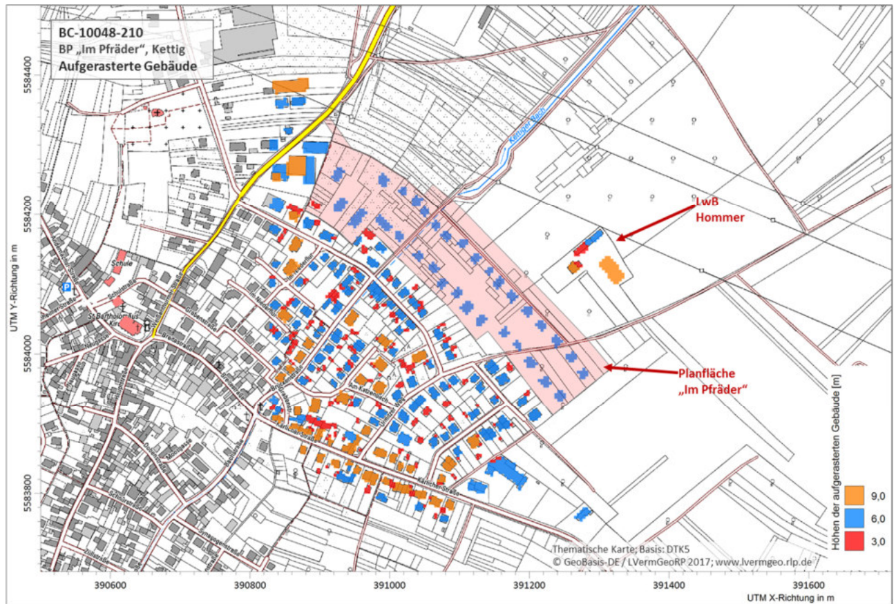
Abbildung 16: Aufgerasterte Gebäude
