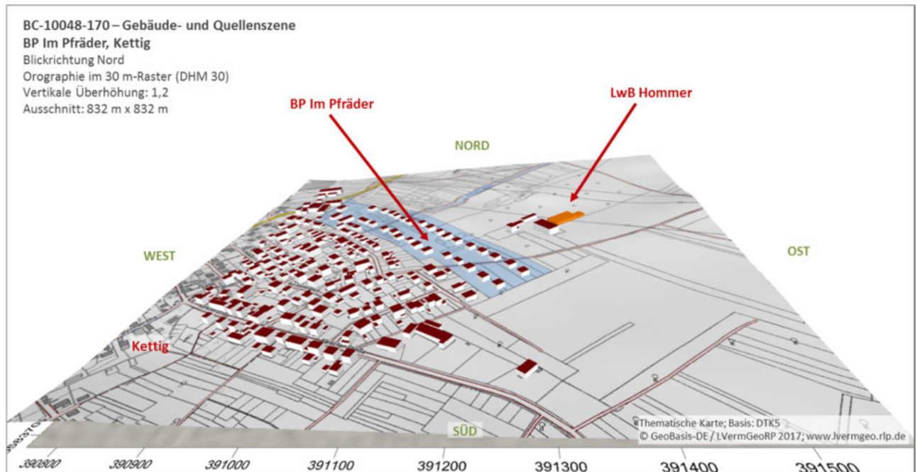
Abbildung 15: 3D-Gebäude-Szene – Blickrichtung West
