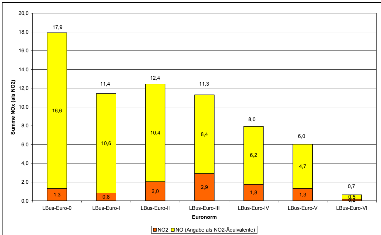
Abb. 28 Mittlere \text{NO}_x -Emissionsfaktoren für Linienbusse im Innerortsverkehr in g/km, HBEFA 3.1
