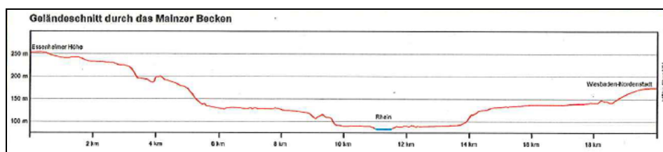
Abb. 11 Geländeschnitt Mainzer Becken von der Essenheimer Höhe bis Wiesbaden-Nordenstadt
