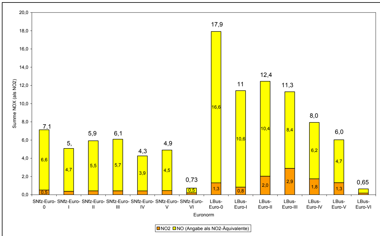
Abb. 23 Durchschnittliche Stickoxid-Emissionsfaktoren innerorts für schwere Nutzfahrzeuge und Linienbusse in g/km
