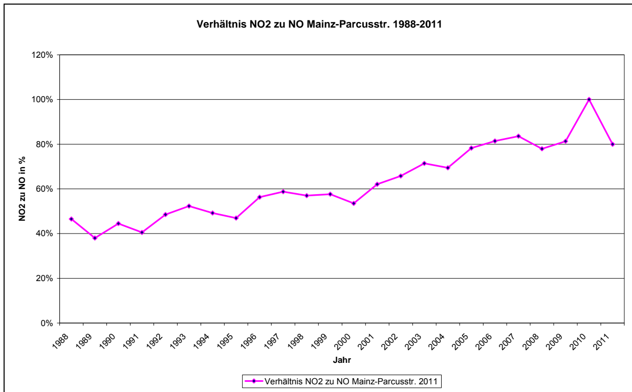
Abb. 15 NO 2 / NO - Verhältnis an der Messstation Mainz-Parcusstr. im Zeitraum 1988-2011
