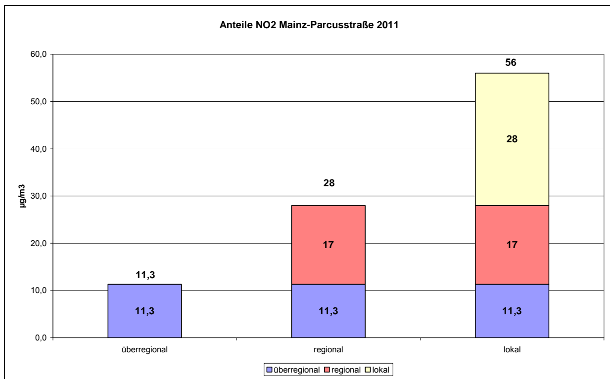
Abb. 17 Zusammensetzung der NO 2 -Belastung in Rheinland-Pfalz, in Mainz und an der Messstation Mainz-Parcusstraße im Jahr 2011 in µg/m 3
