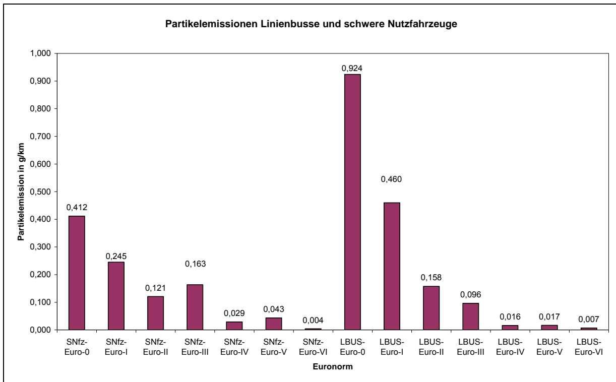
Abb. 26 Durchschnittliche Partikel-Emissionsfaktoren innerorts für schwere Nutzfahrzeuge und Linienbusse in g/km
