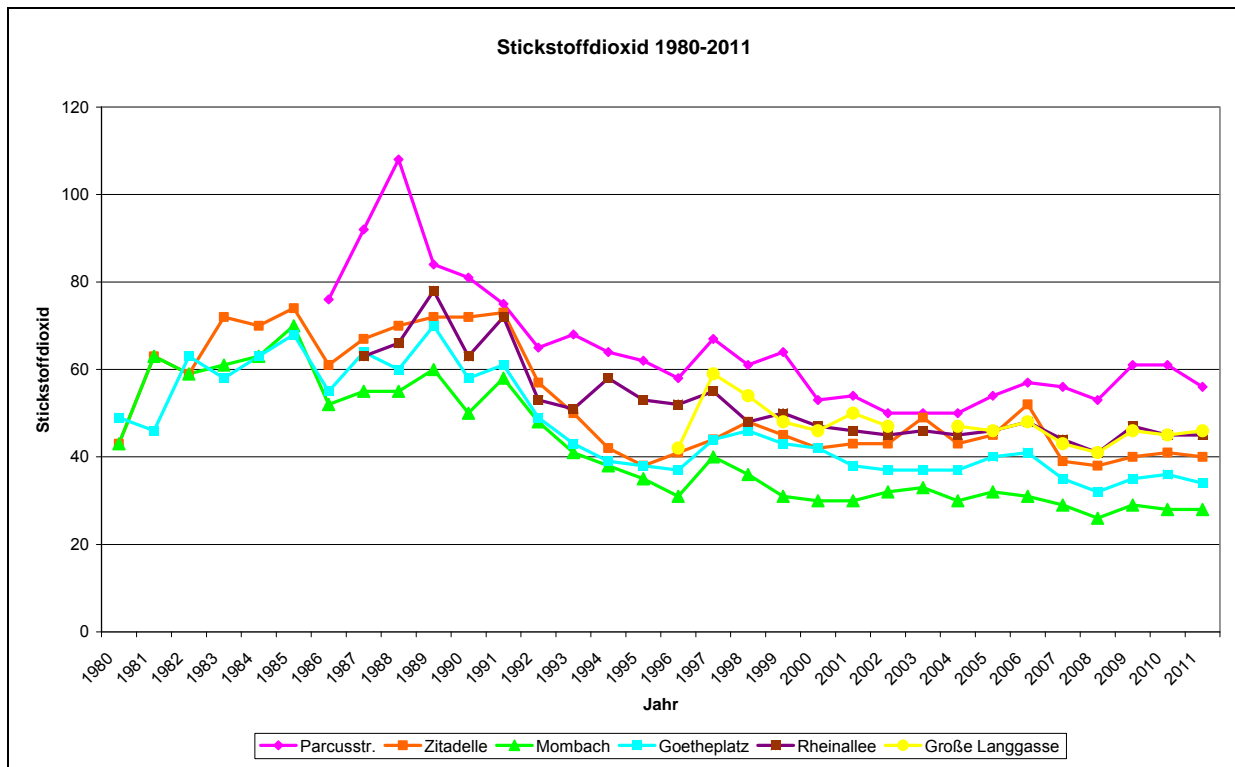
Abb. 14 Langfristige Entwicklung der Stickstoffdioxidkonzentration in Mainz im Zeitraum 1980-2011 in \mu\text{g}/\text{m}^3
