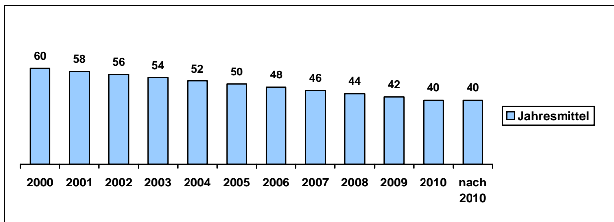
Abb. 2 Immissionswerte für Stickstoffdioxid ( \text{NO}_2 ) in \mu\text{g}/\text{m}^3
