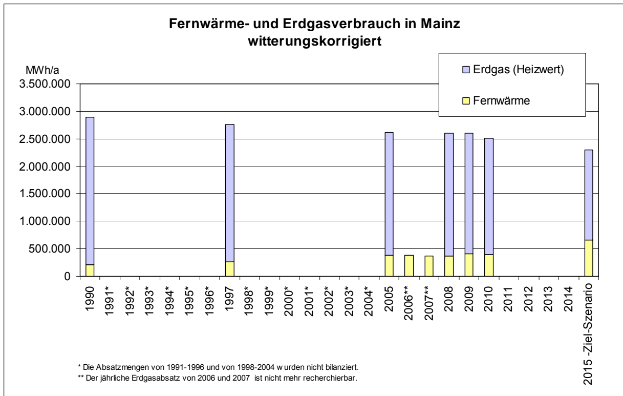
Abb. 30 Fernwärme- und Erdgasverbrauch in Mainz
