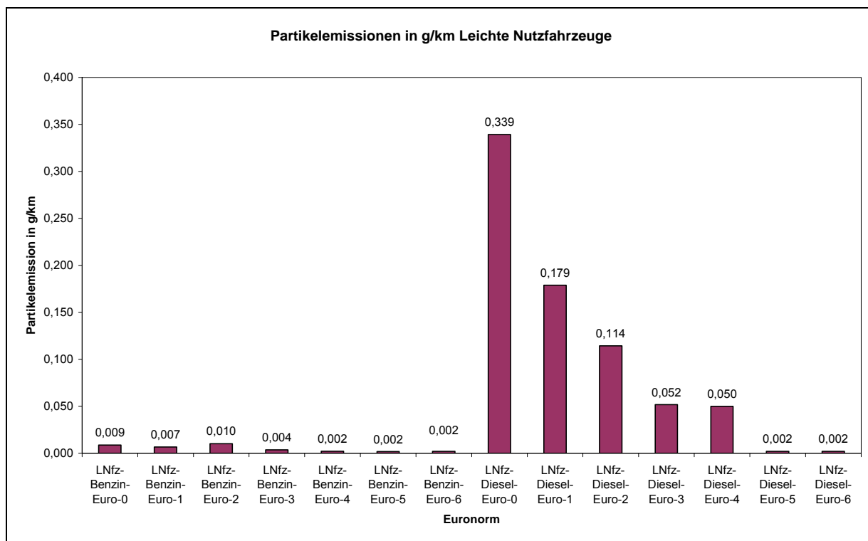
Abb. 25 Durchschnittliche Partikel-Emissionsfaktoren innerorts für leichte Nfz in g/km
