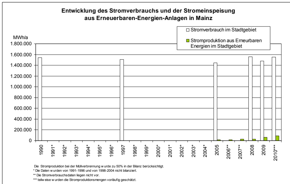
Abb. 33 Entwicklung des Stromverbrauchs und der Stromerzeugung aus erneuerbaren Energiequellen in Mainz
