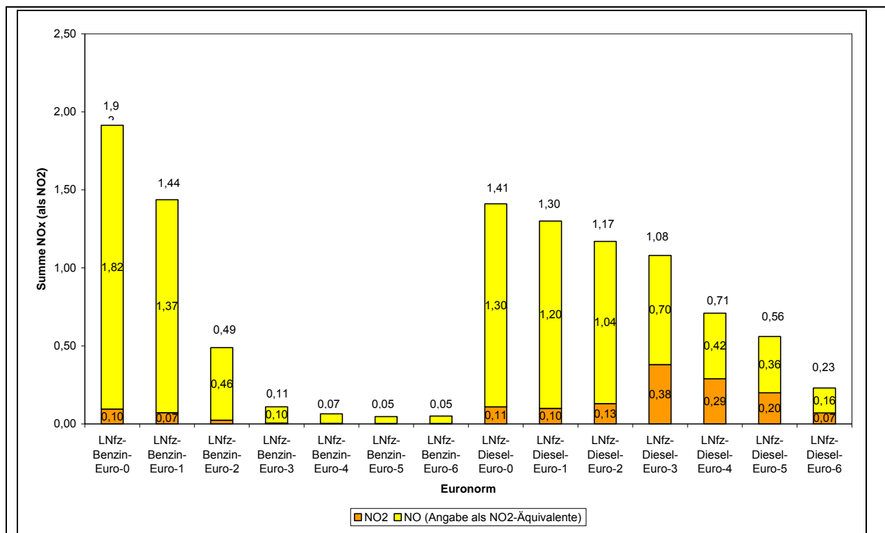
Abb. 22 Durchschnittliche Stickoxid-Emissionsfaktoren innerorts für leichte Nfz in g/km
