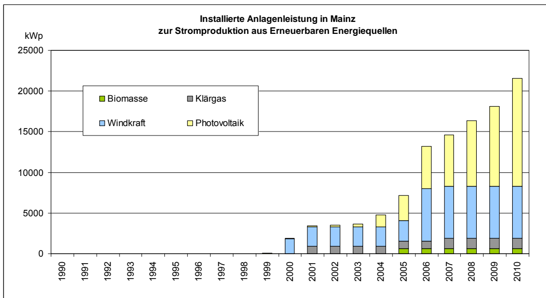
Abb. 32 Installierte Leistung zur Stromproduktion aus erneuerbaren Energiequellen In Mainz
