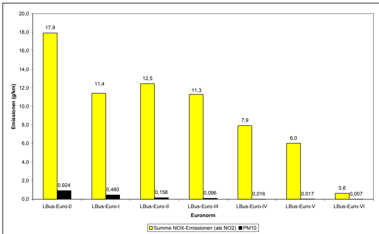
Abb. 34 Durchschnittliche Emissionsfaktoren für Linienbusse im Innerortsverkehr in g/km, HBEFA 3.1
