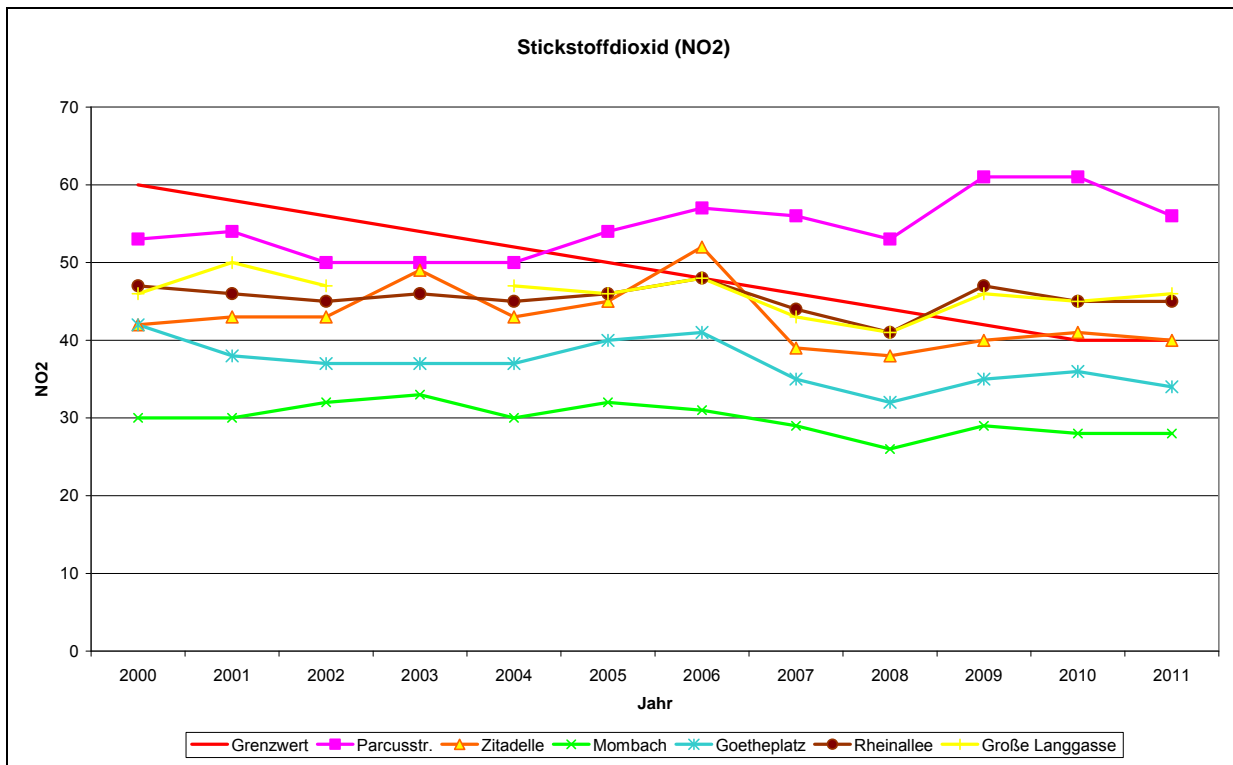
Abb. 13 Entwicklung der Stickstoffdioxidkonzentration in Mainz im Zeitraum 2000-2011 in \mu\text{g}/\text{m}^3
