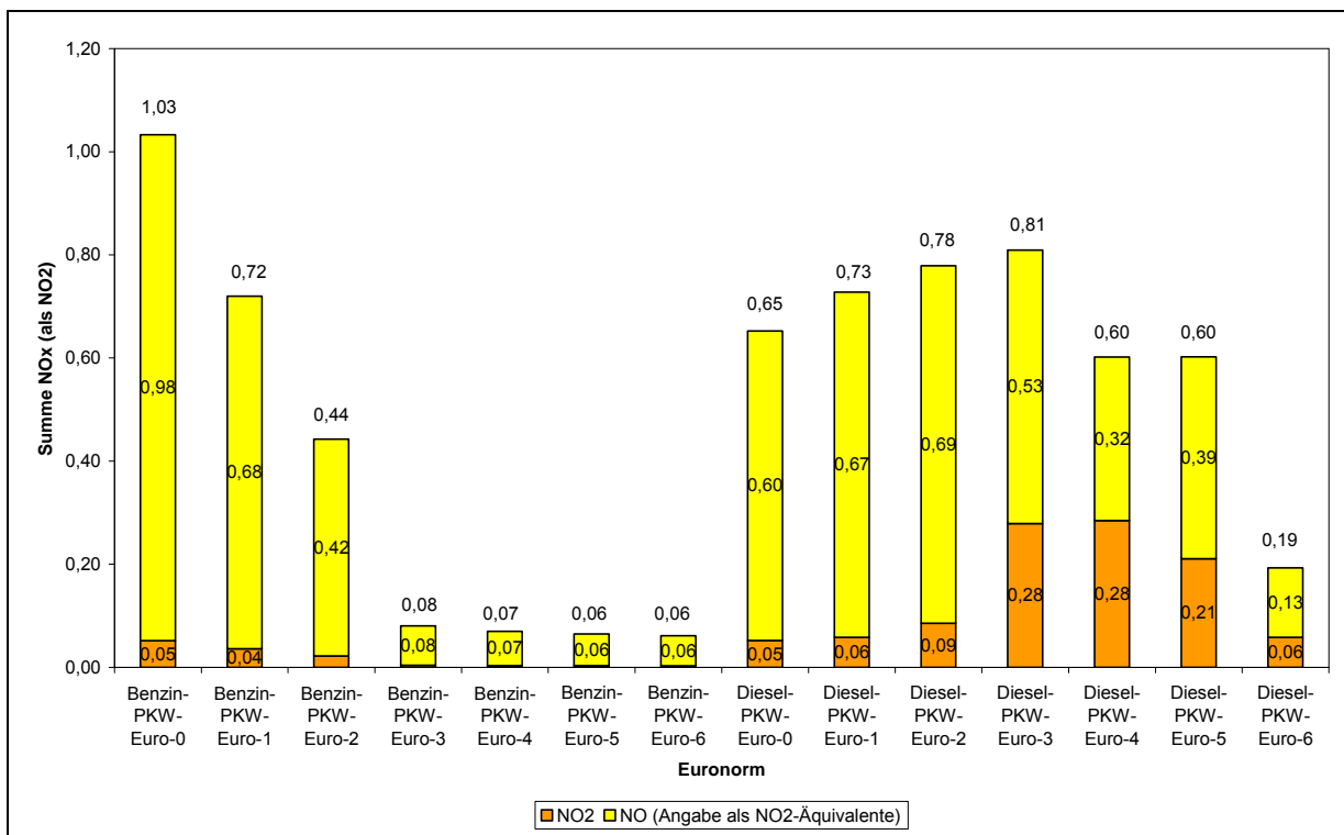
Abb. 21 Durchschnittliche Stickoxid-Emissionsfaktoren innerorts für PKW in g/km
