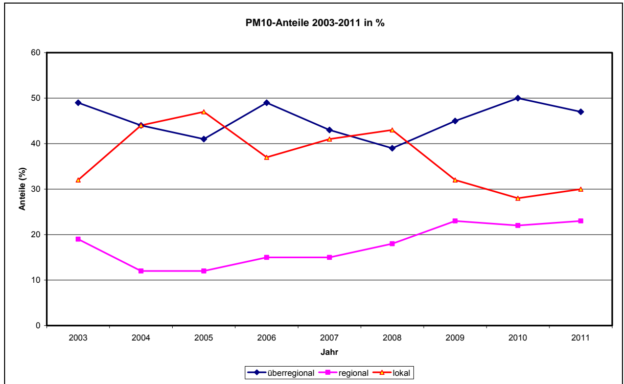
Abb. 18 Entwicklung der überregionalen, regionalen und lokalen Anteile der PM10-Feinstaubbelastung an der Messstation Mainz-Parcusstraße im Zeitraum 2003-2011
