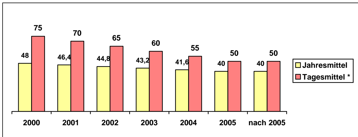
Abb. 1 Immissionswerte für PM10-Feinstaub in \mu\text{g}/\text{m}^3
