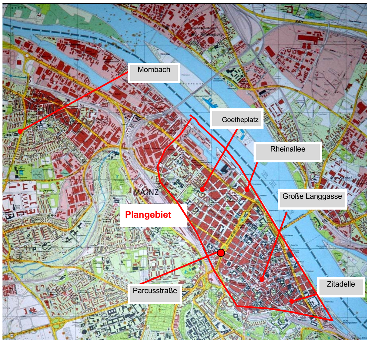
Abb. 3 Plangebiet Mainz mit den Messtationen für PM10-Feinstaub- und Stickstoffdioxid (NO 2 )
