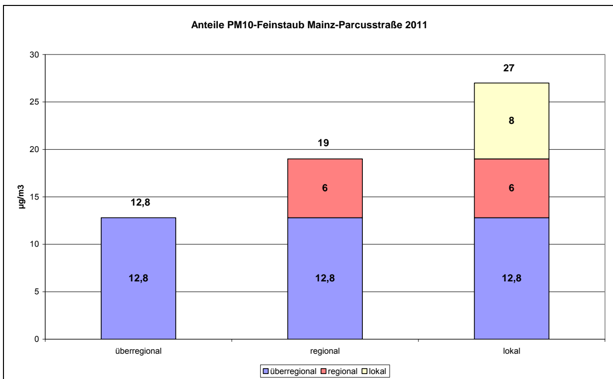
Abb. 16 Zusammensetzung der PM10-Feinstaubbelastung in Rheinland-Pfalz, in Mainz und an der Messstation Mainz-Parcusstraße im Jahr 2011 in µg/m 3
