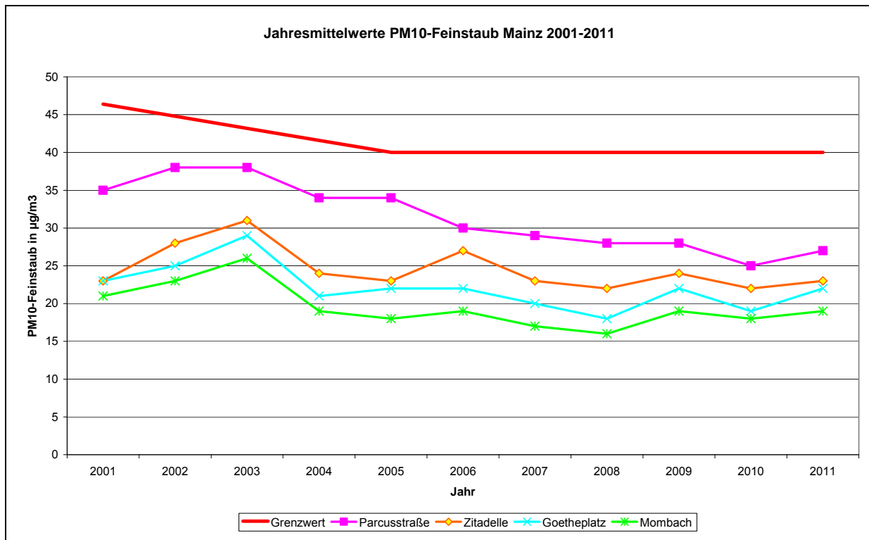
Abb. 12 Verlauf der PM10-Feinstaub-Jahresmittelwerte in Mainz im Zeitraum 2001 bis 2011 in \mu\text{g}/\text{m}^3
