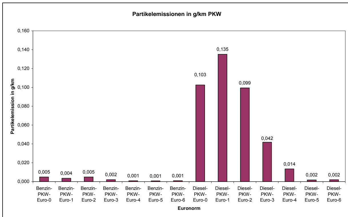
Abb. 24 Durchschnittliche Partikel-Emissionsfaktoren innerorts für PKW in g/km
