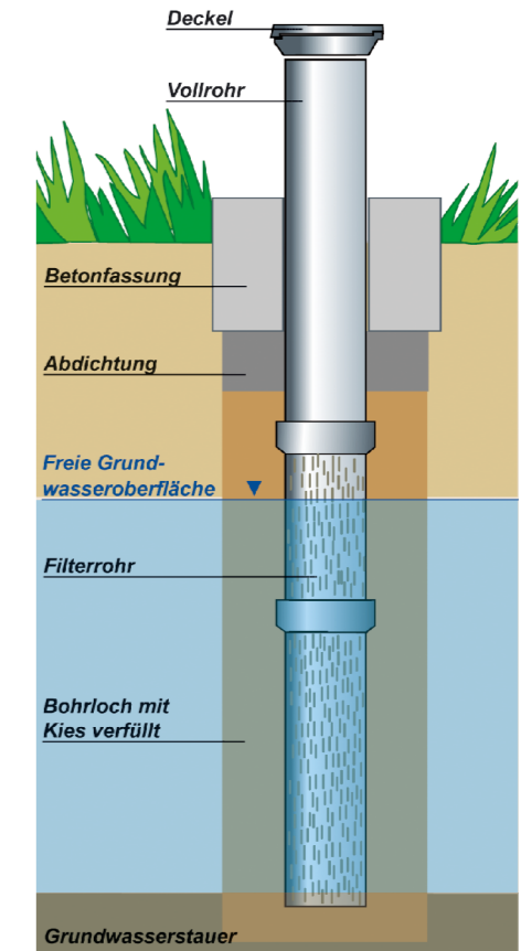
Grundwassermessstelle (Beobachtungsrohr)
