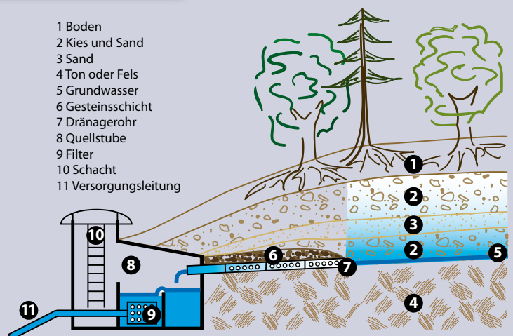
Quellfassung zur Trinkwassergewinnung
