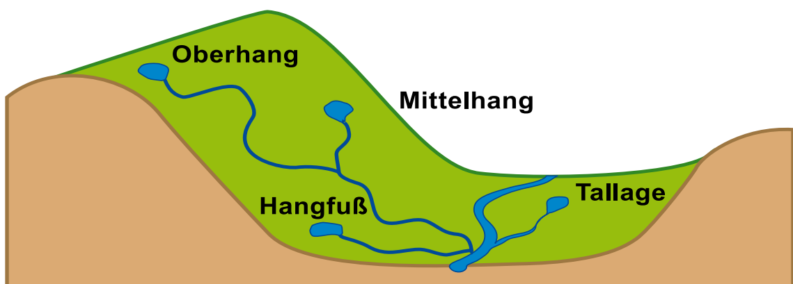
Darstellung von Quellen verschiedener Hanglagen.
