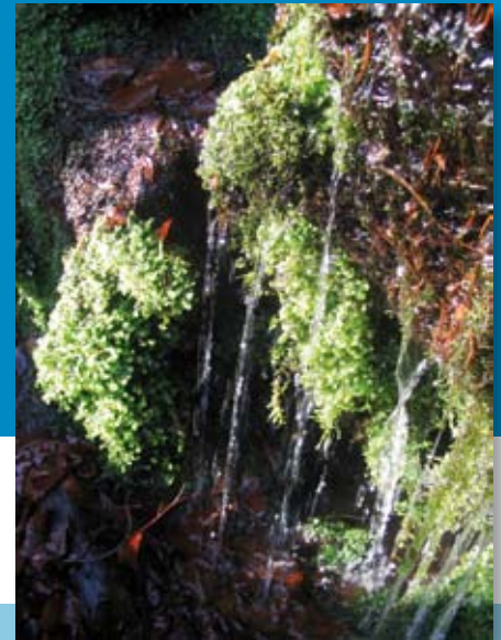
Rieselfluhr, moosbewachsenes Holz/Felsen
