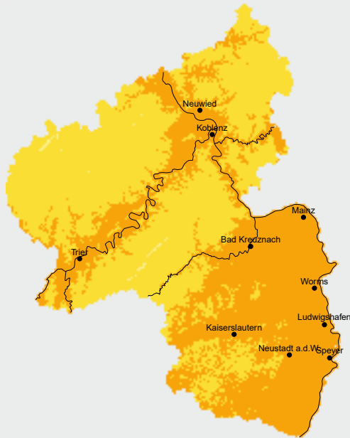
Mitteltemperatur (°C)
