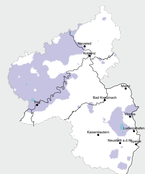
Abweichung Niederschlag (%)
